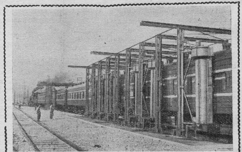
Краснодарский край. На вагонном участке станции Адлер Северо-Кавказской железной дороги успешно прошла испытания и сдана в эксплуатацию вагономоечная машина, изготовленная на Армавирском заводе железнодорожного машиностроения. Стационарная вагономоечная машина, предназначенная для наружной механизированной обмывки пассажирских вагонов, в течение одного часа обрабатывает два состава по 14—16 вагонов в каждом.
