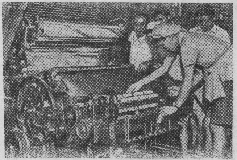
Китайская Народная Республика Коллектив хлопчатобумажной фабрики Цинфэн в городе Уси, центре хлопчатобумажной промышленности провинции Цзянсу, создал новую прядильную машину. Агрегат объединил пять производственных процессов в один. Время обработки сырья сократилось с 24 часов до 5 минут.
