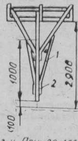
Рис. 4 Прицеп крайних сеялок
