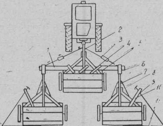
Рис. 1 Общий вид бесцепочного агрегата
