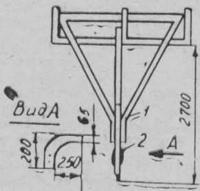
Рис. 3 Прицеп средней сеялки
