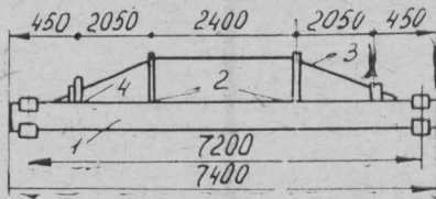
Рис. 2 Тяговый брус бесцепочной сеялки
