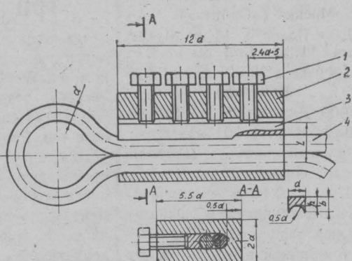
Тросовый замок: 1-болт, 2-корпус, 3-уплотнитель, 4-трос.
