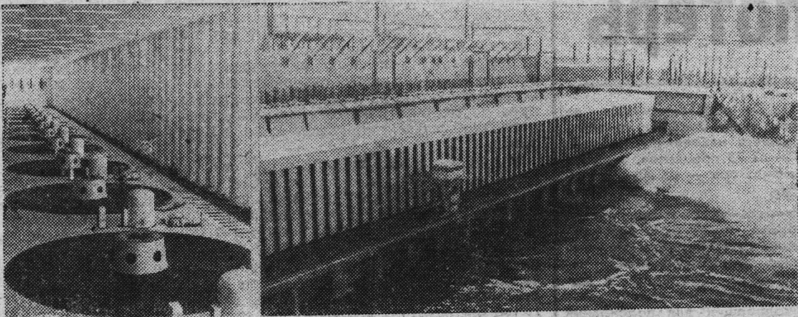
Асуанский гидроэнергетический комплекс — символ современного Египта. На снимках: машинный зал ГЭС; здание ГЭС.
