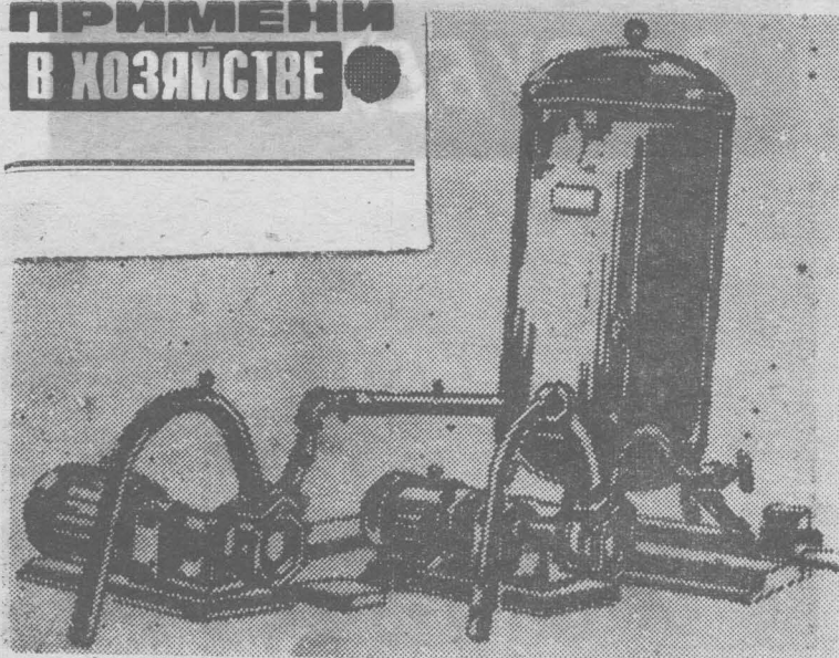
ВОДОПОДЪЕМНАЯ УСТАНОВКА
