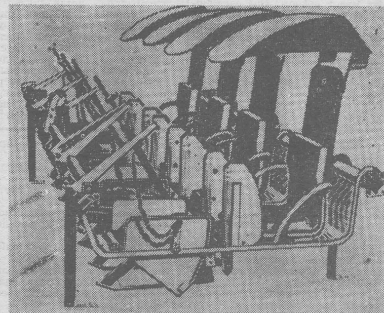
АГРЕГАТ «ПОЛЫЛЬЩИЦА»
