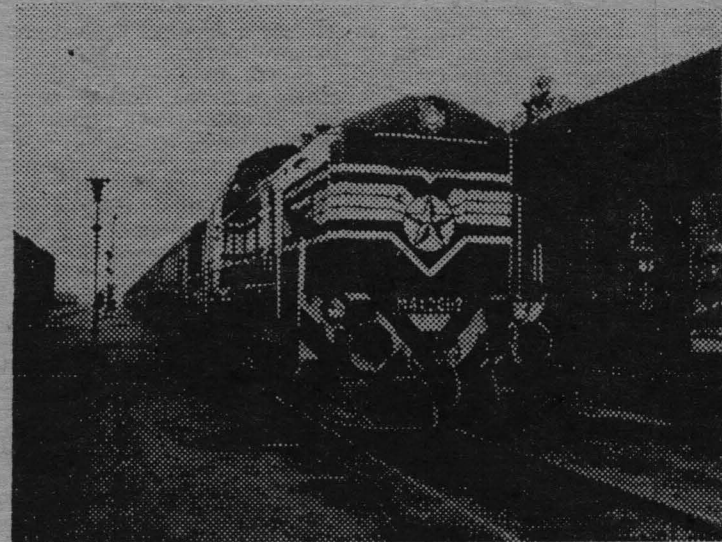
На трассе Будапешт—Сегед проходит испытание первый дизель-гидравлический локомотив типа М-41. Мощность нового локомотива 1200 л. с., скорость — 100 км в час. Он будет использован как для пассажирских, так и для грузовых составов.
