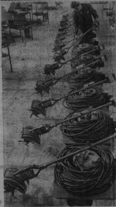
На Ленинградском экспериментальном заводе сельскохозяйственного машиностроения начал серийный выпуск электромотыг «ЭМ-12а» для обработки почвы в теплицах и парниках. Вес мотыги 7 килограммов, а вместе с электродвигателем — 65. В час ею можно обработать на глубину 10 сантиметров 150 квадратных метров почвы.
