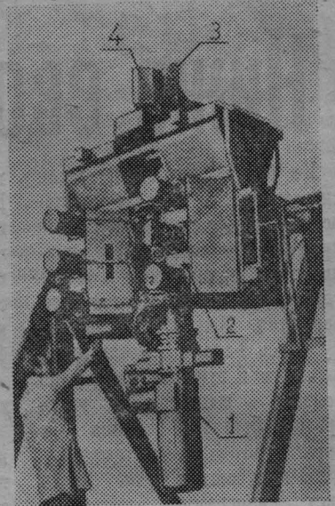
Комплекс научной аппаратуры станции «Протон». 1 — спектрометр электронов (СЭЗ-12); 2 — ионизационный калориметр; 3 — гамма-телескоп (ГГ-1); 4 — спектрометр зарядов частиц малых энергий (СЭЗ-1); Фотохроника ТАСС.
