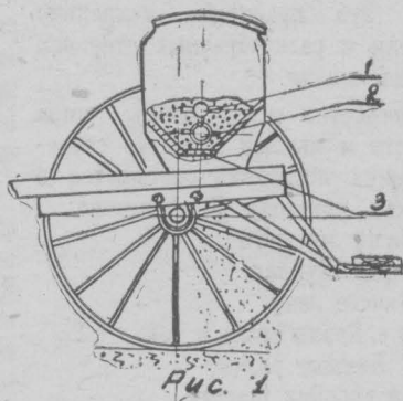
Схема работы сеялки изображена на рис. № 1.
