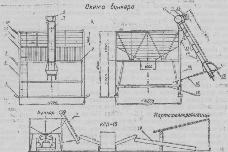
Схема установки картофелесортировального пункта с бункером
