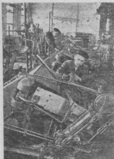
ЛАТВИЙСКАЯ ССР. Лиепайский завод сельскохозяйственного машиностроения приступил к серийному производству жаток-сноповалок модернизированной конструкции. На снимке: сборка жаток.
