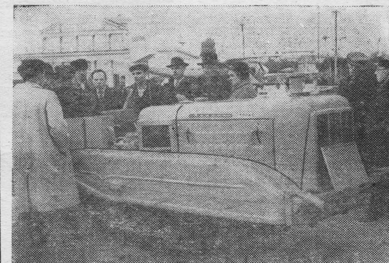
Москва. На Выставке достижений народного хозяйства СССР демонстрируется садово-виноградный трактор Липецкого тракторного завода «Т-50А», снабженный электрогидравлической системой дистанционного управления. Она позволяет управлять трактором по радио на расстоянии до 200 метров и по кабелю на расстоянии в 20 метров.
