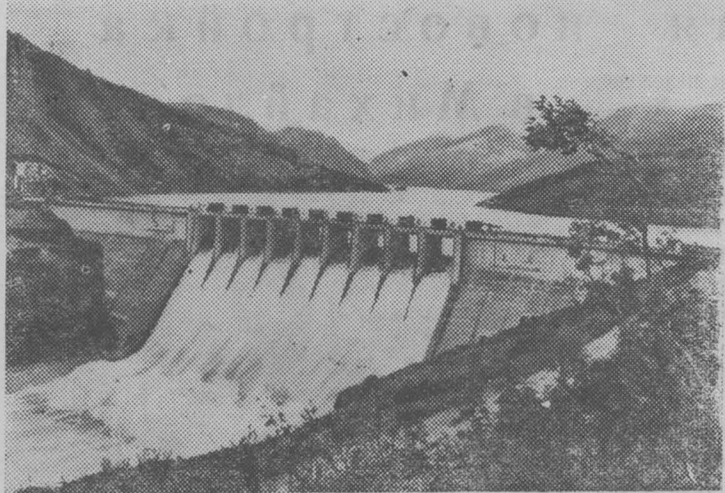
Народная Республика Болгария. На юге страны в горах Восточные Родопы построено одно из крупнейших гидротехнических сооружений Болгарии «Студен кладенец». Строители гидроузла «Студен кладенец» перекрыли русло горной реки Арда плотной длиной 338 метров и высотой 72,5 метра и создали водохранилище длиной 29 километров. Здесь построена гидроэлектростанция мощностью 60.000 киловатт.
