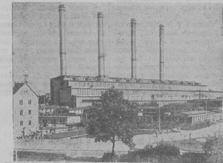
Германская Демократическая Республика. Общий вид электростанции, Фокероде. На электростанции, построенной в годы народной власти, работает 12 агрегатов общей мощностью 384 тысячи киловатт.
