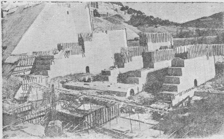
Народная Республика Болгария. В Ихтиманской околии сооружается водохранилище «Тополница». Его длина 12 километров, емкость 140 миллионов кубометров воды. Создание водохранилища даст возможность оросить 400 тысяч декаров земли (декар — 1/10 гектара).
