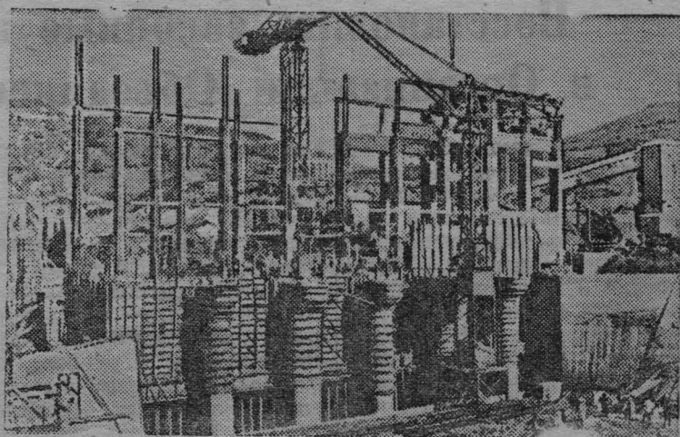
Грузинская ССР. Строительство Гуматской ГЭС-2 вступило в предпусковой период. Ускоренными темпами ведутся бетонные и монтажные работы. На стройке широко развернулось социалистическое соревнование в честь XX съезда КПСС.
