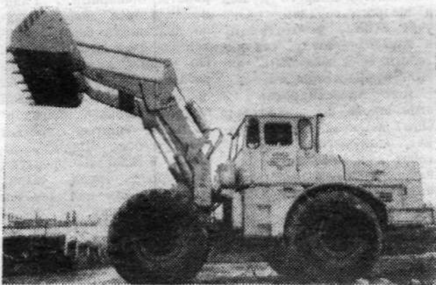
Белорусская ССР. К серийному выпуску навесных колесных погрузчиков для сельского хозяйства (на снимке) приступил завод «Могилевсельмаш». Агрегат разработан на базе трактора К-701. Его грузоподъемность — 4 тонны. В этом году будет выпущено 600 таких машин.
