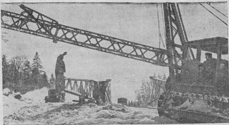
Приморский край. Через тайгу, хребты Сихотэ-Алиня и горные реки прокладывают линию электропередачи монтажники Приморского участка управления «Дальэнергомонтаж». Новая линия рассчитана для передачи тока напряжением 220 тысяч вольт на расстояние 355 километров от Сучанской ГРЭС до поселка Го-
