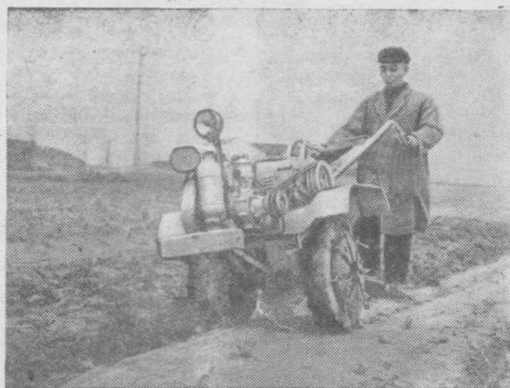
Китайская Народная Республика. В этом году шанхайские заводы намеряют выпустить около 800 небольших универсальных тракторов. Первый трактор был изготовлен на заводе Хунсин («Красная звезда»). На тракторе установлен двигатель мощностью в 4 лошадиных силы.
