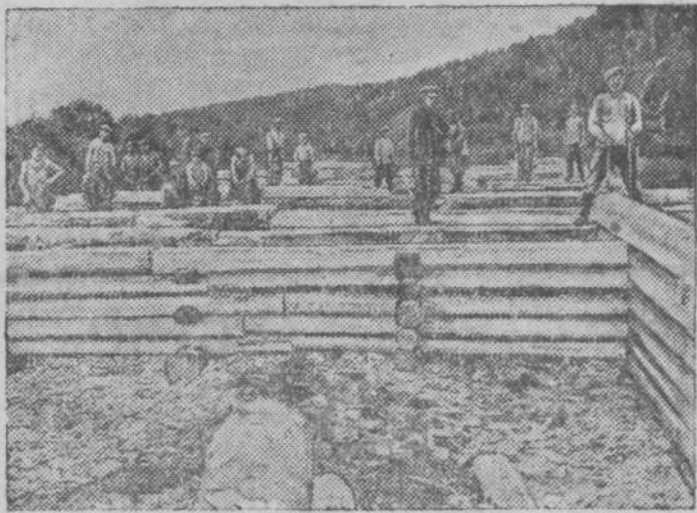
Крапивинская ГЭС. Плотники на рубке ряжа.
