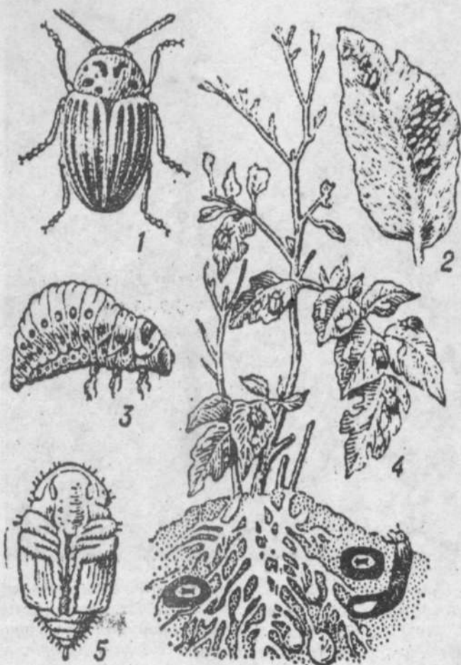
Колорадский картофельный жук: 1 - жук; 2 - кладка яиц; 3 - личинка; 4 - личинки и жуки, объедающие листья картофеля; 5 - куколка.
