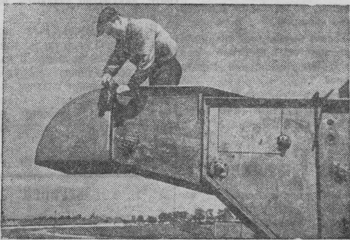
Комбайнер Расшеватской МТС (Ордженикидзевский край) А. К. Простасов, работа на комбайне, удлинил соломотранспортер и молотилку, добавил два лагера и это позволило сохранить часть зерна, которое обычно выходило с соломой при работе комбайна на уборке.
