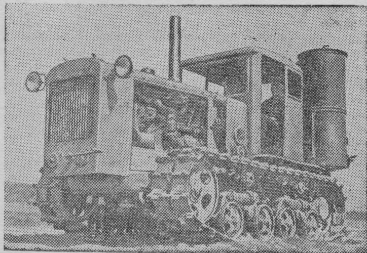
НА СНИМКЕ: Газогенераторный трактор ХТЗ. А. Иоселевича (Союзфото).
