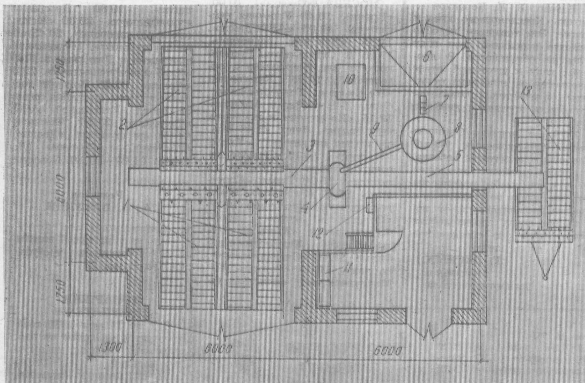
Схема кормоцеха Петуховского комплекса: 1 — приемное устройство для сенажа и соломы; 2 — приемное устройство для силоса; 3 — ленточный транспортер; 4 — измельчитель-смеситель ИСК-30; 5 — скребковый транспортер ТК-5; 6 — завальная яма для концентратов; 7 — нория; 8 — бункер Б-6; 9 — шнековый дозатор; 10 — электрокалорифер; 11 — электропульт управления; 12 — пульт управления; 13 — мобильный кормораздатчик КТУ-10.
