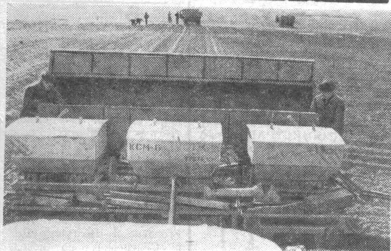
РЯЗАНСКАЯ ОБЛАСТЬ. На полях колхоза «Красная заря» Рязанского района проходят испытания шестирядной картофелесажалки (на снимке). КСМ-6 создана конструкторами Рязанского производственного объединения по машинам для возделывания картофеля и корнеплодов.
