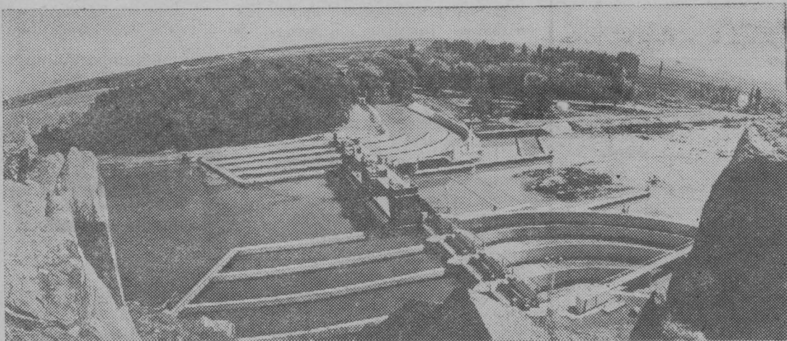
КИРГИЗСКАЯ ССР. Чумышская плотина на реке Чу—полностью автоматизированный гидротехнический узел, который дает воду тысячам гектаров хлопковых плантаций Киргизии и Казахстана.
