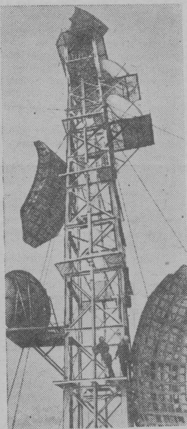
КИРГИЗСКАЯ ССР. Мощная радиорелейная станция, связывающая молодой город Чолпон-Ата на побережье высокогорного озера Иссык-Куль с Останкинским телецентром, позволяет жителям этого отдаленного района республики смотреть цветные передачи из Москвы.
