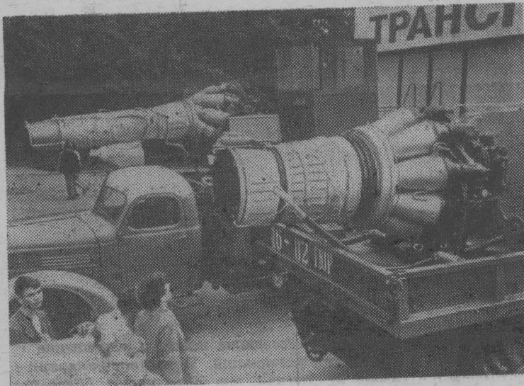
НА СНИМКЕ: мощный аэрозольный генератор МАГ-3 (на переднем плане). (Фотохроника ТАСС).
