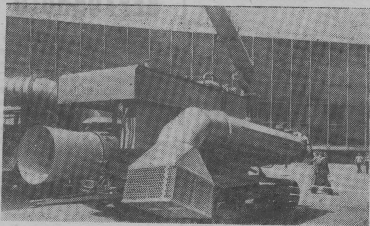
НА СНИМКЕ: дальнеструй. ДМ-1000 «Нептун III». Она новая дождевальная машина предназначена для полива сп-
