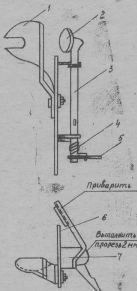
1. Схема реконструкции высаживающего аппарата для высадки мелких клубней: 1 - ложечка; 2 - пластина зажима; 3 - зажим; 4 - пружина; 5 - рычаг; 6 - диск; 7 - ушко.
