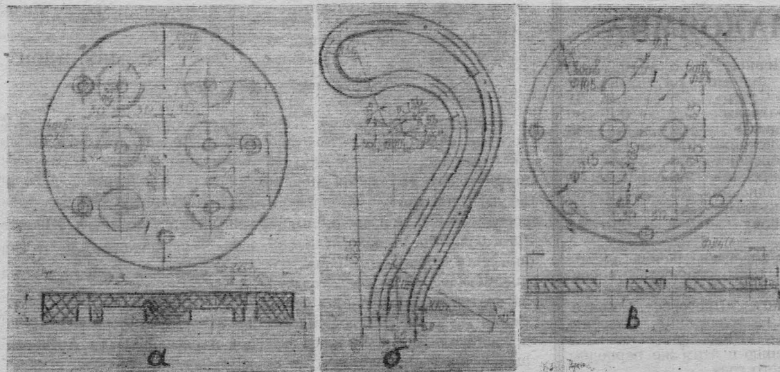
Рис. 1. Детали блока электронагревательных элементов: а — клеммная панель; б — нагревательный элемент; в — фланец.
