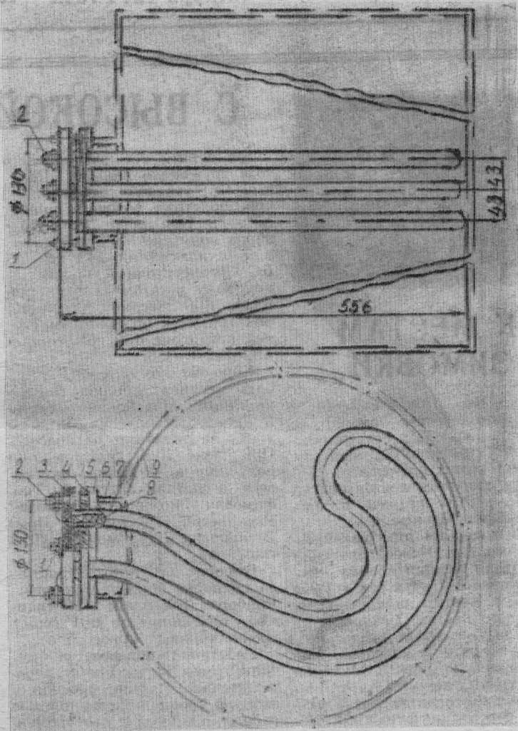
Рис. 2. Блок электронагревательного элемента в сборе: 1 и 2 — болты; 3 — клеммная панель; 4 — фланец блока; 5 — существующий фланец водонагревателя; 6 — кольцо Рашига; 7 — электронагревательный элемент; 8 — спираль из нихромовой проволоки; 9 — корпус (показан условно).
