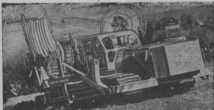
Новую технику для осушительных работ применяют мелiorаторы народного предприятия «Мелиораторносоюз» в Карл-Маркс-Штадте (ГДР). На этом снимке вы видите высокопроизводительный агрегат. С его помощью можно прокладывать пластмассовые и керамические дренажные трубы без выемки почвы. Фото АДН-ТАСС
