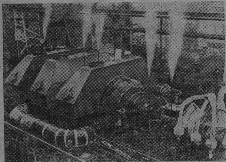
ЛЕНИНГРАД. Большую трудовую победу одержал коллектив Металлического завода — закончена сборка и успешно проведены испытания паровой однофазной турбины мощностью 300 тысяч киловатт. Это новый вклад ленинградских турбостроителей в успешное завершение второго года семилетки.
