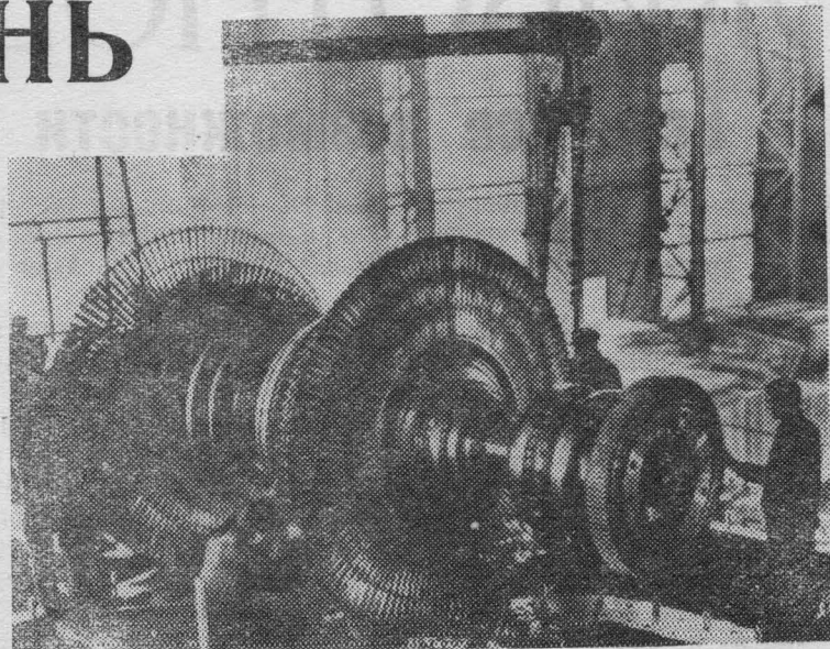
КИТАЙСКАЯ НАРОДНАЯ РЕСПУБЛИКА. На Харбинском заводе турбогенераторов создана первая в стране паровая турбина мощностью 100 тысяч киловатт. На снимке: установка ротора турбины. Фото Цан Лу.
