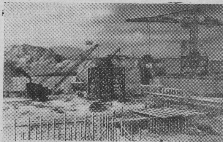
ТАДЖИКСКАЯ ССР. Строители одной из крупнейших в Средней Азии Головной ГЭС отказались от сооружения дорогостоящей бетоновозной эстакады. Вместо нее решено установить два 25-тонных башенных крана. Это намного удешевит и сократит сроки строительства.
