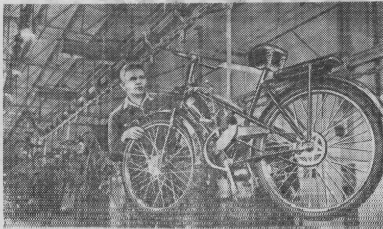
Львов. Мотовелосипеды «В-902», выпускаемые заводом «Металл», снискали заслуженную похвалу у трудящихся страны. Это очень удобная дорожная машина, способная нести на себе груз до 100 килограммов и развивать скорость до 45 километров в час. Она снабжена двухтактным одноцилиндровым двигателем мощностью в одну лошадиную силу. Расход горючего — два литра на 100 километров пробега.
