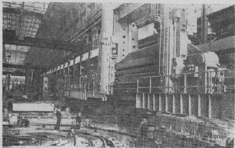
УКРАИНСКАЯ ССР. В гидротурбинном цехе Харьковского турбинного завода монтируется крупный токарно-карусельный станок, на котором можно обрабатывать детали диаметром до 22 метров и весом в сотни тонн. На снимке: монтаж станка-гиганта.
