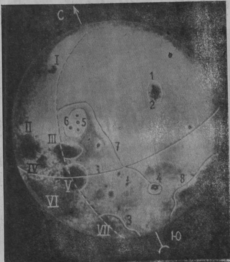
Распределение объектов на невидимой с Земли стороне Луны, выявленных при предварительной обработке фотографий, полученных с борта автоматической межпланетной станции: 1. Большое кратерное море диаметром 300 км—море Москвы; 2. Залив Астронавтов в море Москвы; 3. Продолжение Южного моря на обратной стороне Луны; 4. Кратер с центральной горкой Циолковский; 5. Кратер с центральной горкой Ломоносов; 6. Кратер Жолно-Кюри; 7. Горный хребет Советский; 8. Море Мечты. Сплошная линия, пересекающая схему,—лунный экватор; пунктирная линия—граница видимой и невидимой с Земли частей Луны. Римскими цифрами обозначены объекты видимой части Луны: I—море Гумбольдта; II—море Кризисов; III—море Красное; IV—море Воли; V—море Смита; VI—море Падородия; VII—море Южное.
