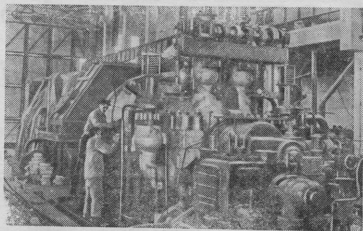
На нефтеперерабатывающем заводе в Узбекской ССР. Фотохроника ТАСС.
