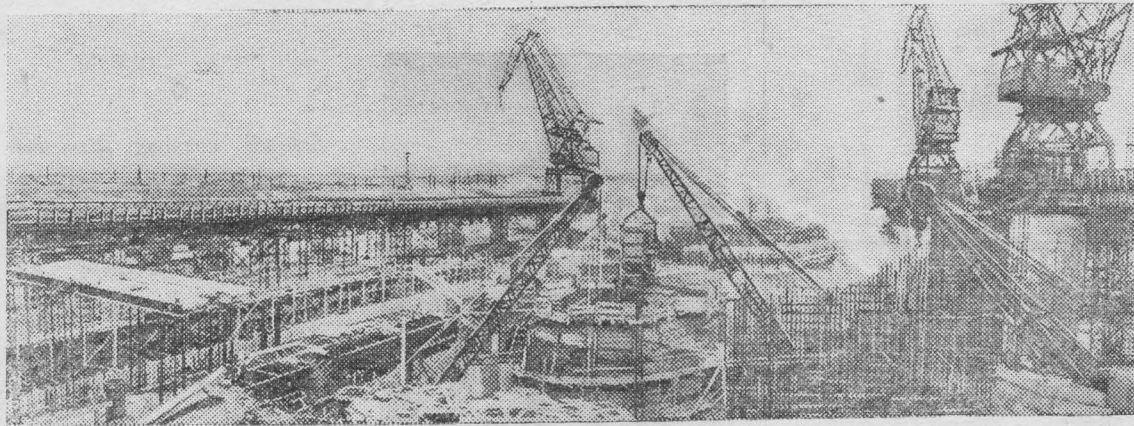
Строительная площадка Иркутской ГЭС на реке Ангаре.
