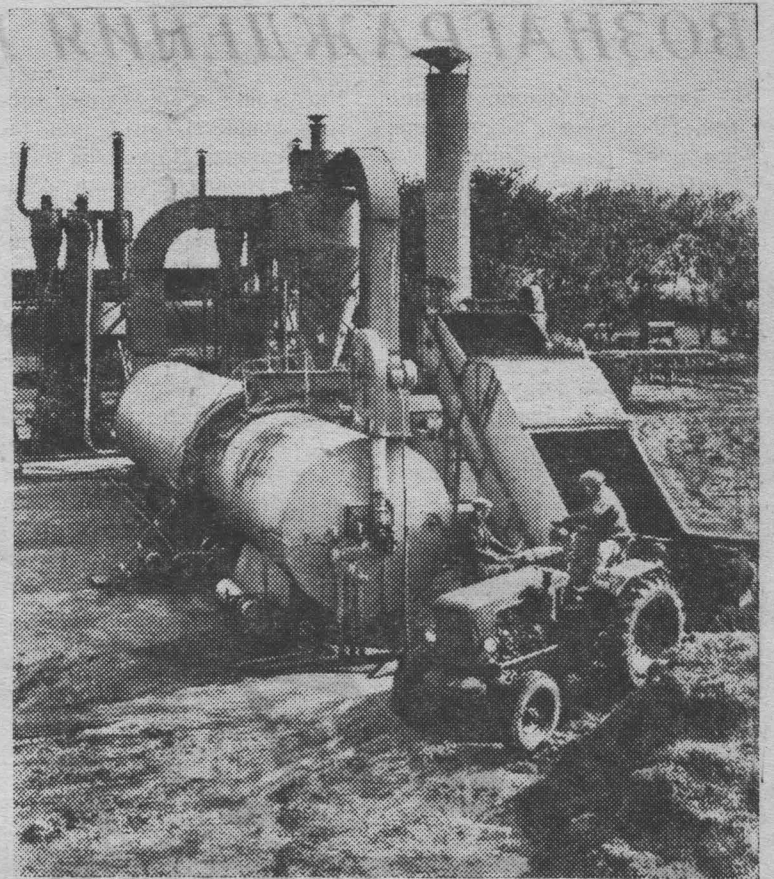
НИКОЛАЕВСКАЯ ОБЛАСТЬ. В колхозе «Родина» Баштанского района идет косовица трав на культурных орошаемых пастбищах. Заработала установка СБ-1,5 по приготовлению витаминно-травяной муки (на снимке). Всею за сезон будет заготовлено 1500 тонн этого ценного гранулированного корма.
