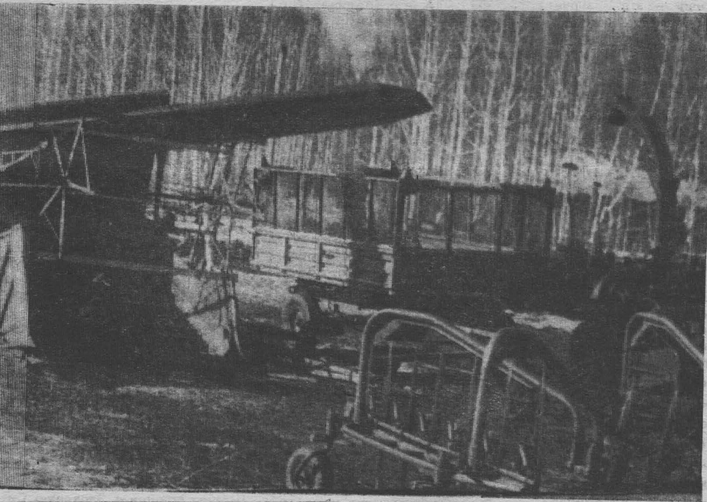
НА СНИМКЕ: НАБОР МАШИН ДЛЯ ПРИГОТОВЛЕНИЯ СЕНАЖА. СИЛОСНЫЙ КОМБАЙН КС-2,6 С ПОДБОРЩИКОМ; ИЗМЕЛЬЧИТЕЛЬ КИК-1.4; ГРАБЛИ РОГАЦИОННЫЕ; ТЕЛЕЖКА ТРАКТОРНАЯ.
