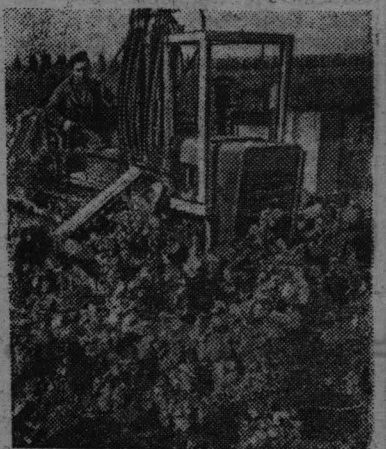
МОЛДАВСКАЯ ССР. По виноградным плантациям движется необычная машина. Внизу рядом с кабиной водителя находится режущий аппарат. Срезанный гроздь по транспортеру подается в бункер.
