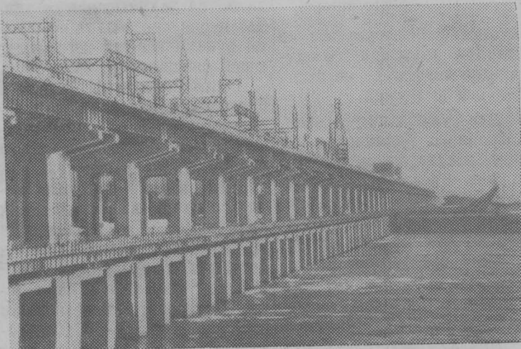
Сталинградская ГЭС. Ее последний 21-й по счету гидроагрегат недавно вступил в строй действующих. Фото С. Курнина.
