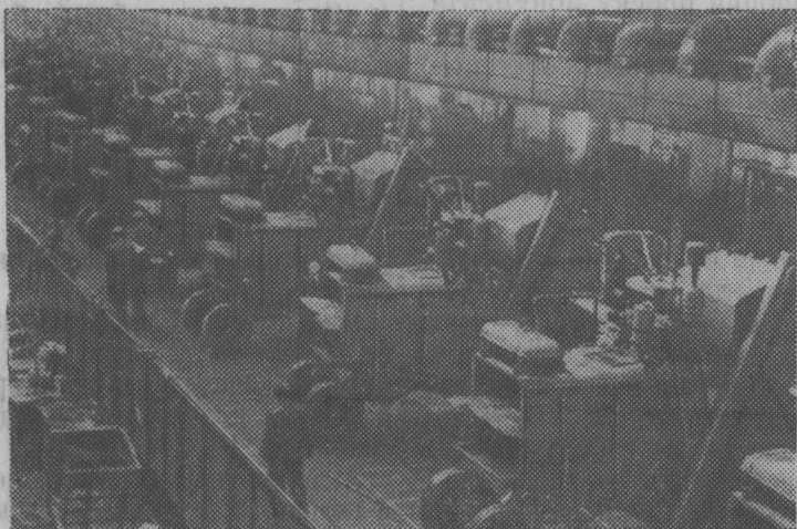
Ростов-на-Дону. Выпуск самоходных комбайнов с начала семилетки на заводе „Ростсельмаш“ возрос на 46,2 процента. Комбайн „СК-3“ прочно вошел в сельскохозяйственное производство. Эта машина получила признание не только в нашей стране, но и за ее пределами. Но скоро на главном конвейере завода появятся новые, еще более совершенные машины—самоходный комбайн „СК-4“. Производительность его на 25 процентов выше, чем у комбайна „СК-3“.
