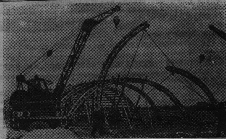
Латвийская ССР. В колхозе «Саркана звайгзне» Елгавского района строится телятник нового типа—из сборных железобетонных арок. Конструкция телятника весьма проста, сборка каркаса занимает несколько дней. При этом не требуется никакого фундамента. На снимке: сборка нового телятника в колхозе «Саркана звайгзне».
