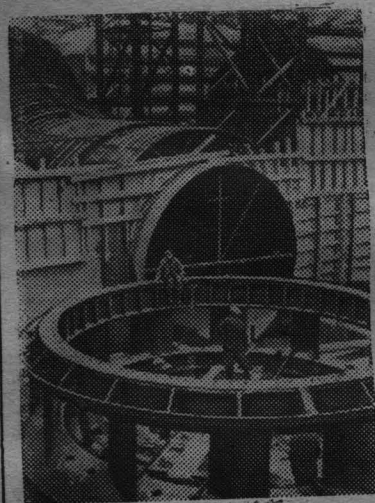
Иркутская область. Строители Братской ГЭС установили в проектное положение статор первого гидроагрегата.
