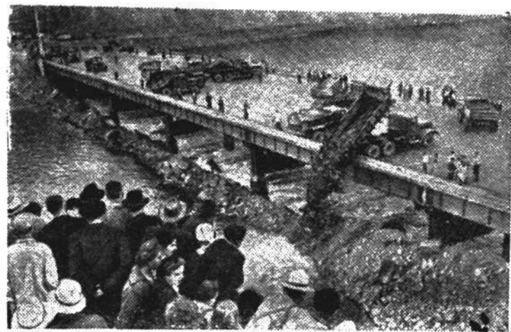
19 июня строители Братской ГЭС закончили перекрытие Ангары.
