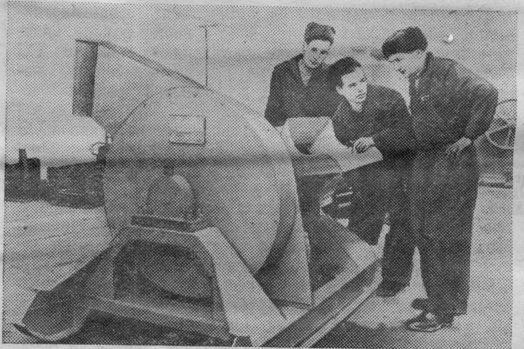
Одесская область. Коллектив Килийского судоремонтного завода сконструировал и построил для колхозов и совхозов района, над которыми шефствует, несколько машин, измельчающих солому на скормливание скоту. Испытания машины показали хорошие результаты.
