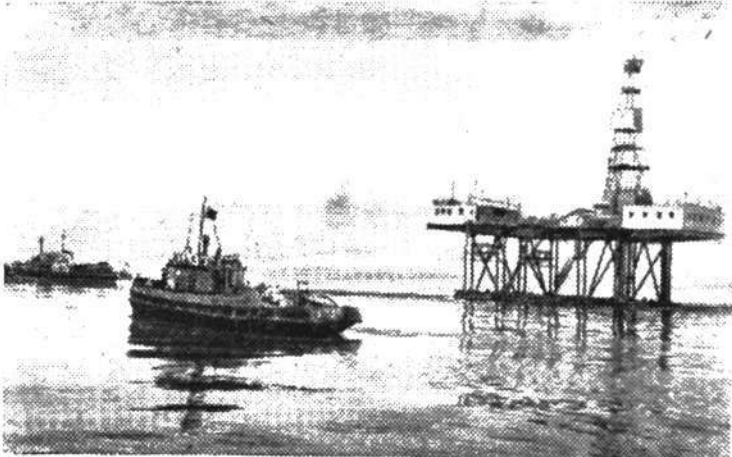
Азербайджанская ССР. В Баку проводится испытание плавучего морского основания, предназначенного для бурения разведочных скважин при глубине моря от 2 до 6,5 метра. Основание представляет собой стальной плавучий остров, состоящий из затопляемого понтона и верхней площадки в 500 квадратных метров, на которой располагаются буровая вышка, необходимое оборудование и жилые помещения. После окончания бурения из понтона выкачивается вода, и остров всплывает на поверхность, готовый к транспортировке в другое место.
